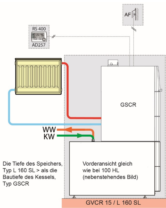
OEnoviaTower Gas GVCR 15, L 160 SL Brauchwasserspeicher Aufstellung L 160 SL nur als Säule, 1,69 m Raumhöhe notwendig
