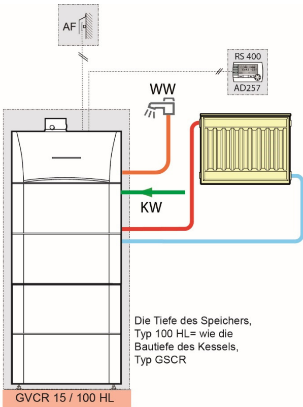
OEnoviaTower Gas GVCR 15, 100 HL Brauchwasserspeicher Aufstellung 100 HL nur als Säule, 1,63 m Raumhöhe notwendig
